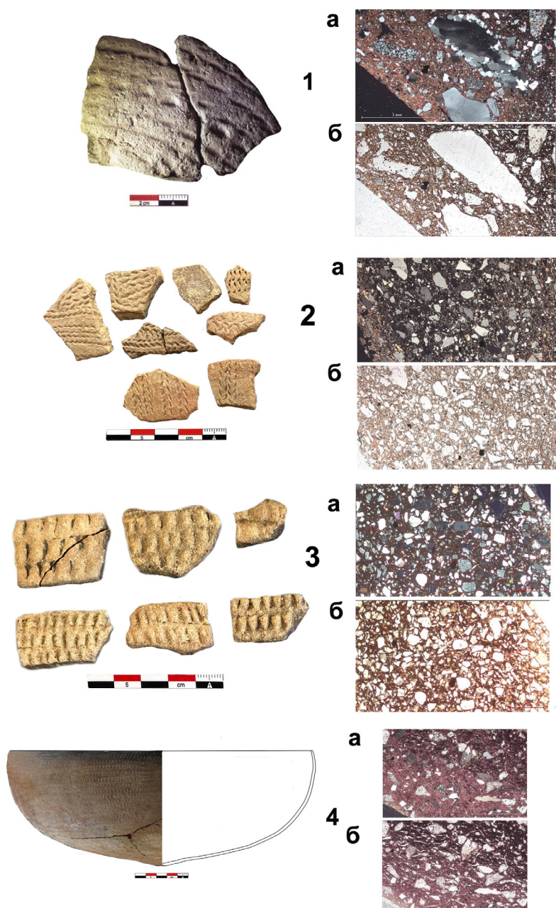
Рис. Микрофотографии типов керамического материала неолитической керамики Ониба: 1 – «грубая» керамика, 2 – «сланцеватая» керамика, 3 – «железистая» керамика, 4 – керамика из захоронения. Прозрачный шлиф с анализатором (а) и без анализатора (б).
