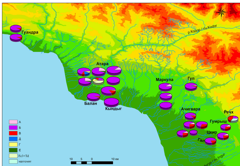
Рис. 1. Локализация исследованных глин: диаметр круга соответствует общему содержанию Fe (мас. %), цвет долей диаграмм – типу группы или уникальной формы по данным мёссбауэровских спектров.
