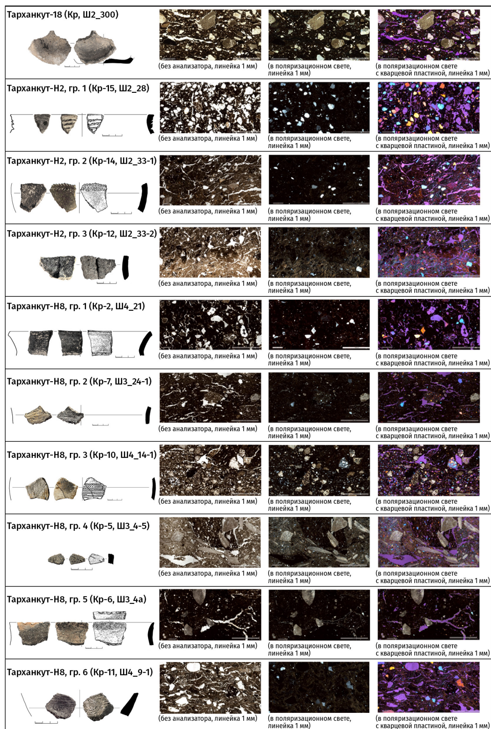
Рис. 2. Результаты петрографического исследования керамики из поселений с «загонами для скота» Т-18, Т-Н2 и Т-Н8 на Тарханкуте (образцы, шлифы и технологические группы), выборочно.
