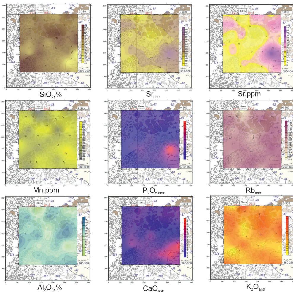
Рис 2. Геохимические карты распределения элементов и антропогенных компонентов по участку опробования на Каратаевском городище.
