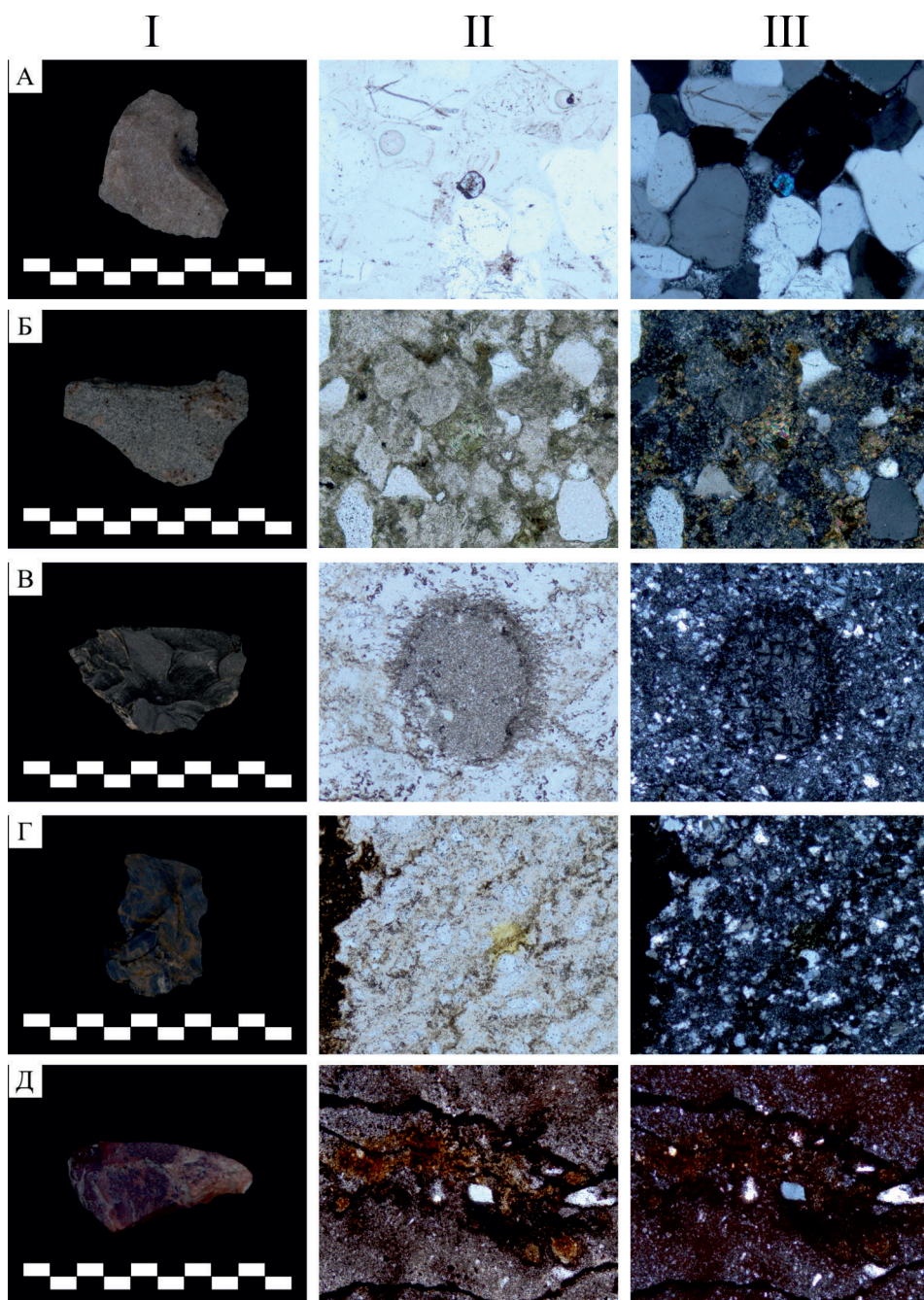
Рис. Некоторые представительные образцы отщепов. I – общий вид образца; II – фрагмент шлифа без анализатора; III – фрагмент шлифа с анализатором. А – кварцевый песчаник; Б – песчаник; В – кремль; Г – яшма; Д – яшмокварцит.
