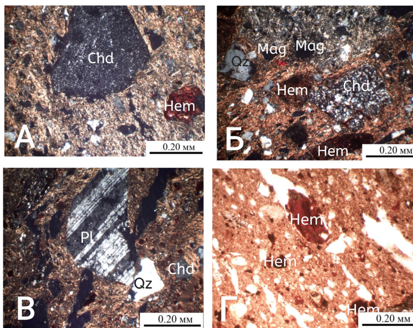
Рис. 2. Микрофотографии керамических изделий: А) угловатый обломок халцедона (Chd) и пылеватое скопление гематита (Hem), фотография в отраженном свете; Б) угловатые обломки кварца (Qz) со ступенчатыми границами, пылеватые скопления гематита (Hem), угловатые и округлые зерна магнетита (Mag), фрагмент халцедона (Chd), фотография при скрещенных николях; В) деформированное зерно олигоклаза (Pl), угловатые фрагменты халцедона (Chd) и кварца (Qz), фотография при скрещенных николях; Г) пылеватые скопления гематита (Hem), фотография в отраженном свете.
