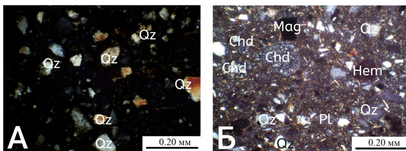
Рис. 3. Микрофотографии глин: А) угловатые зерна кварца (Qz), фото при скрещенных николях; Б) зерна кварца (Qz) со ступенчатыми границами, округлые зерна халцедона (Chd), деформированное зерно олигоклаза (Pl), прямоугольное зерно магнетита (Mag), овальное зерно гематита (Hem), фото в отраженном свете.
