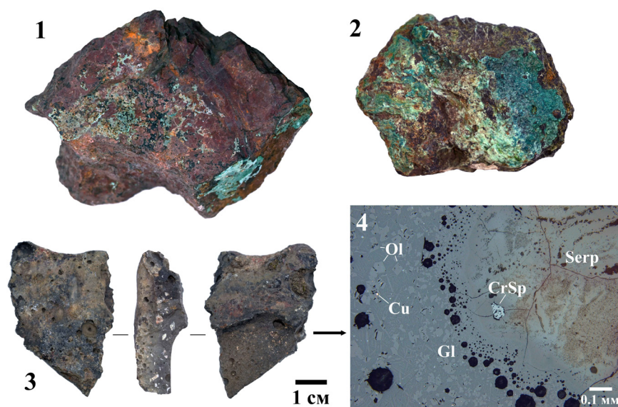
Рис. 1. Фрагменты горных пород с медной минерализацией и металлургического шлака из подъемных сборов с территории укрепленного поселения Княженское 17. 1 – гематит-кварцевая порода, шифр КП-25 б/н руда; 2 – медно-магнетитовая руда, шифр КП-25 б/н1; 3 – фрагмент лепешковидного металлургического шлака, шифр КП-25/176; 4 – микроструктура металлургического шлака: частично оплавленный реликт серпентинита (Serp) с включением хромшпинелида (CrSp) и мелкие капли меди (Cu) в основной массе шлака, представленной новообразованными кристаллами оливина (Ol) и стеклом (Gl); шифр КП-25/176; фото в отраженном свете.
