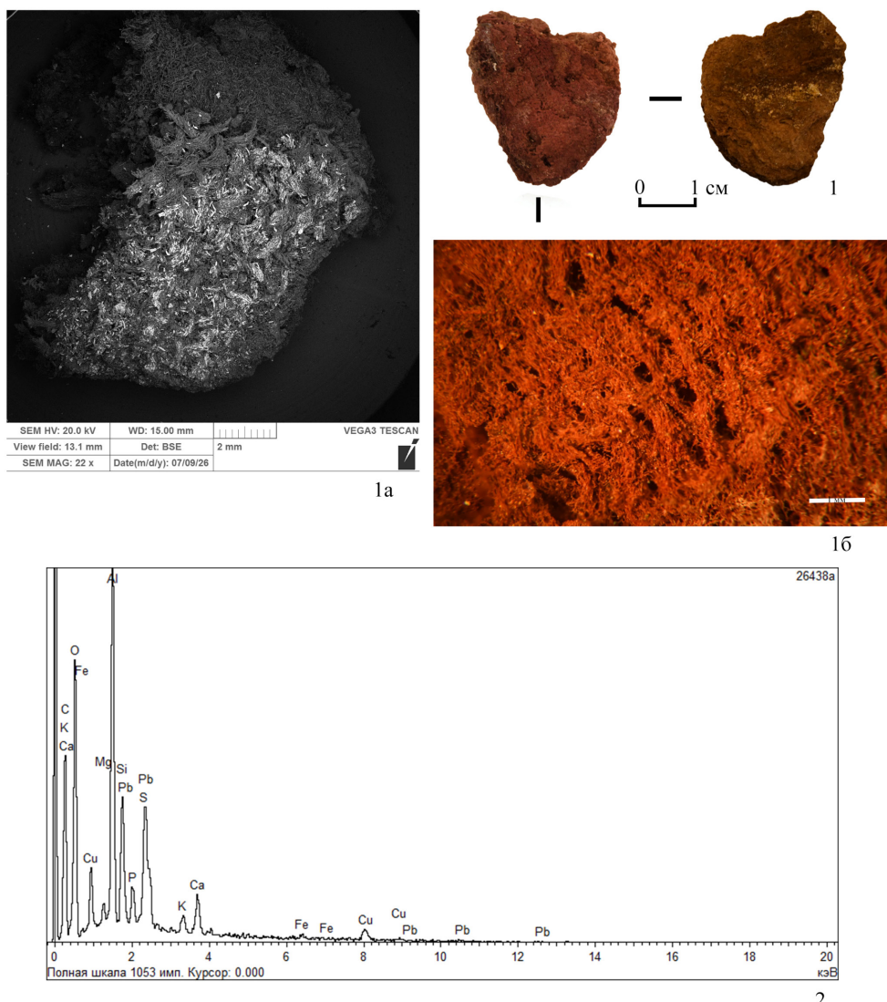
Рис. 2. Могильник Магнитный, курган 21, могильная яма 1. 1, 1а – фрагмент текстиля, 1б – фрагмент текстиля (увел. 16×); 2 – энергодисперсионный спектр текстиля.
