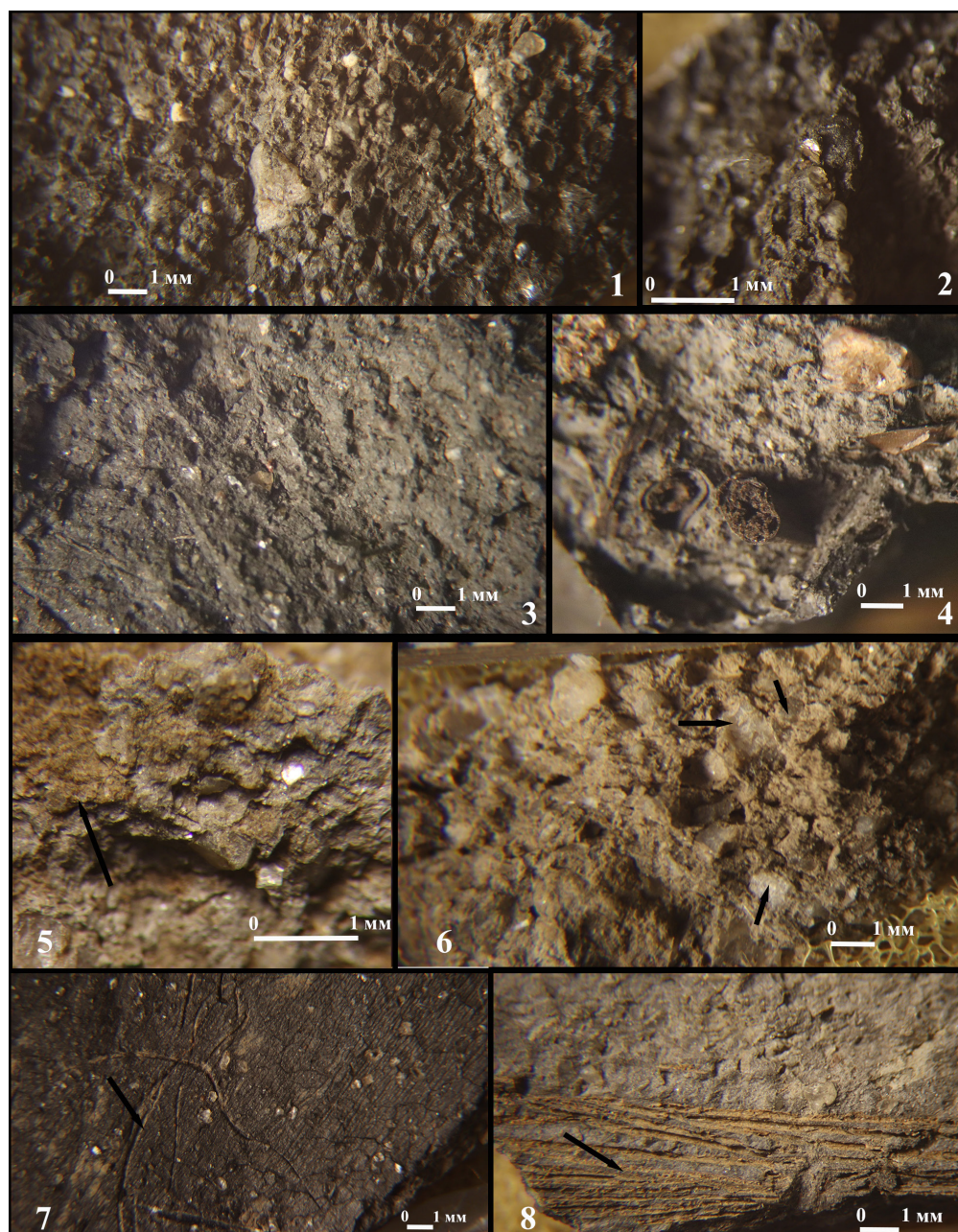
Рис. Фото образцов. 1, 2 – эталоны, изготовленные из глины, отобранной вблизи стоянки Михеевская 2; 3, 4 – эталоны, изготовленные из илистой глины, отобранной вблизи стоянки Михеевская 2; 5 – излом сосуда с органическим раствором; 6 – излом сосуда с примесью кварцевого песка; 7 – поверхность сосуда с отпечатками шерсти; 8 – излом сосуда с отпечатками шерсти.
