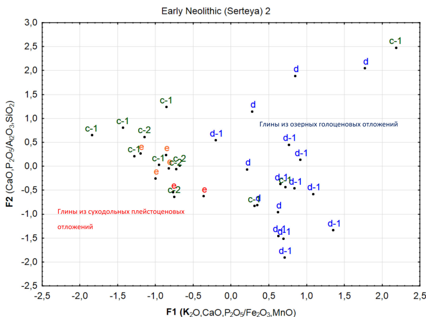
Рис. Статистический анализ результатов XRF образцов сосудов раннего неолита (для каждого образца указаны фазы керамики раннего неолита (по Долбунова и др., 2023).
