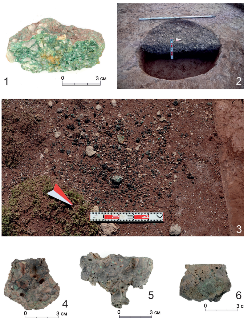
Рис. 1. Поселения Коктас 1 (раскоп 1): 1. – Малахит из помещения «А»; 2 – разрез ямы с рудой, расположенной к югу от помещения «В»; 3 – Скопление шлака в юго-западной части раскопа 1; 4 – Шлак KTS-1; 5 – Шлак KTS-3; 6 – Шлак KTS-2.
