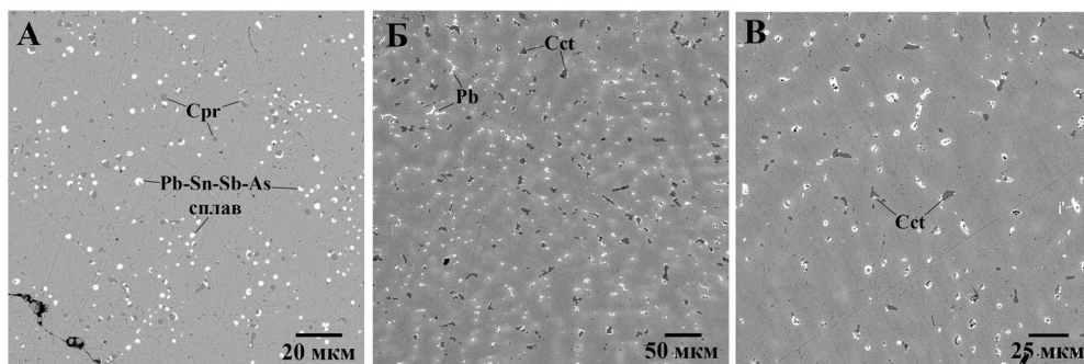
Рис. 1. Микроструктуры металлических котлов. А – котел 1; Б – котел 2; В – котел 3. Обозначения минералов: Срг – куприт, Ссг – халькозин. Фото в отраженных электронах.
