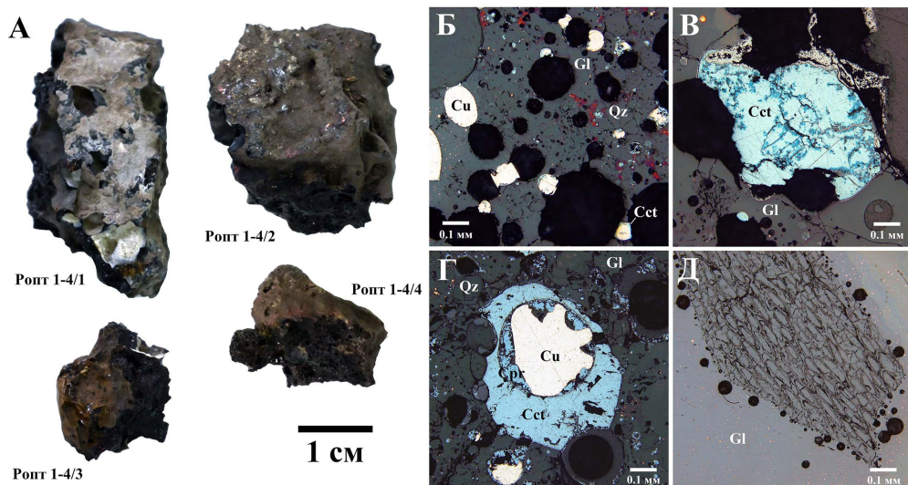
Рис. 3. Металлургические шлаки с поселения Роптанка II. А – общий вид, Б–Д – фото полированных аншлифов в отраженном свете: Б – зерна кварца (Qz) и капли меди (Cu) в матрице стекла шлака (Gl), образец Ропт 1-4/4; В – включения халькозина (Cct) в стекле шлака), образец Ропт 1-4/4; Г – капля меди с каймой из новообразованных куприта (Cpr) и халькозина), образец Ропт 1-4/1; Д – реликт окремненной древесины), образец Ропт 1-4/1.
