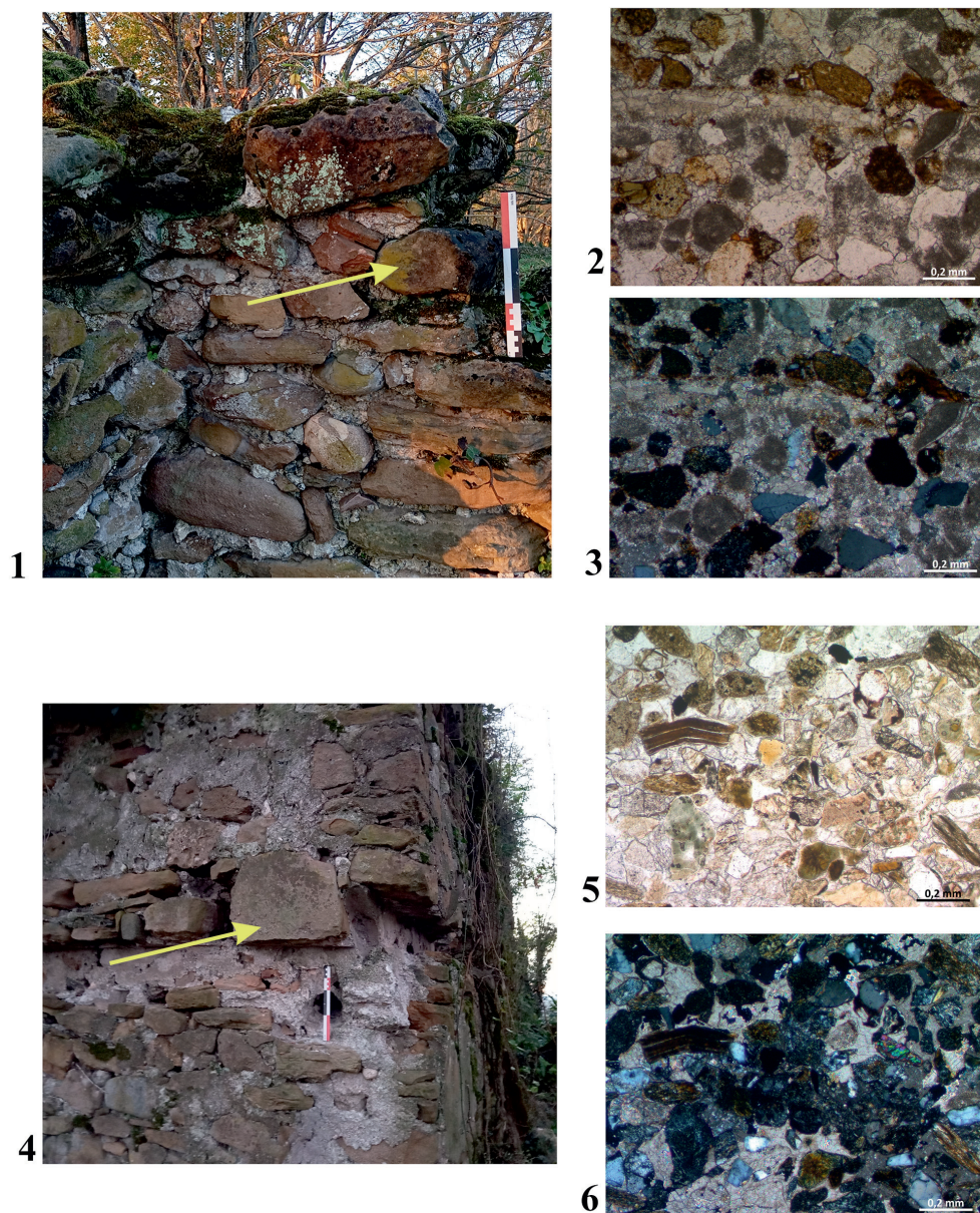
Рис. 1. Исследуемые камни из кладок храма и башни на Маркульском городище: 1 – местоположение камня в храме; 2 – камень из кладки стены храма без анализатора; 3 – камень из кладки стены храма с анализатором; 4 – местоположение камня в башне Алахаш-Абаа; 5 – камень из кладки в башне Алахаш-Абаа (без анализатора); 6 – камень из кладки в башне Алахаш-Абаа (с анализатором).
