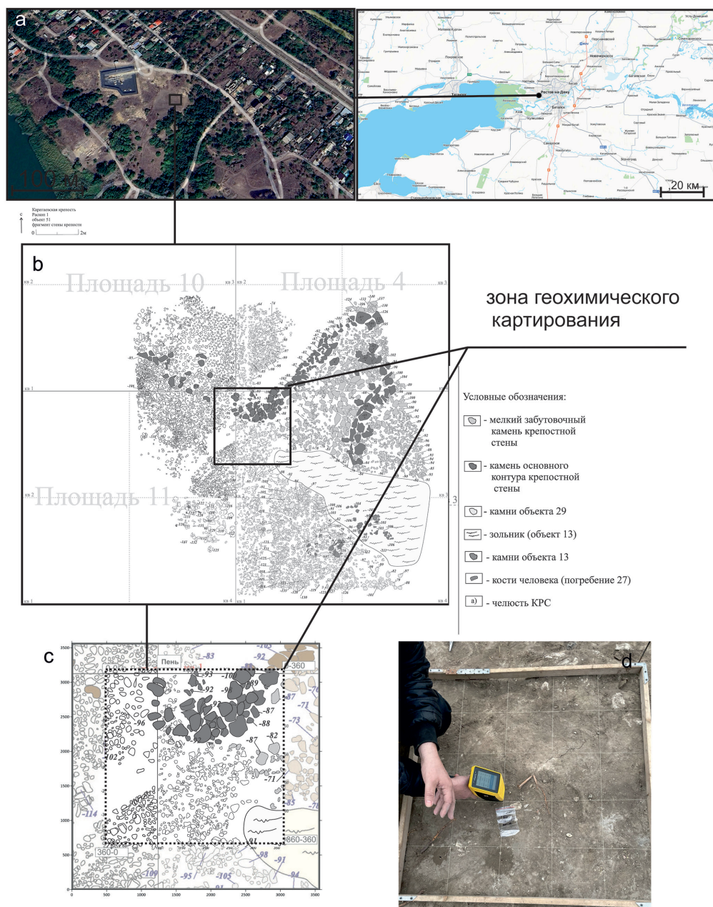
Рис 1. Расположение памятника «Каратаевское городище»: (а), план раскопа (б), зона геохимического опробования (с), проведение измерений (д).
