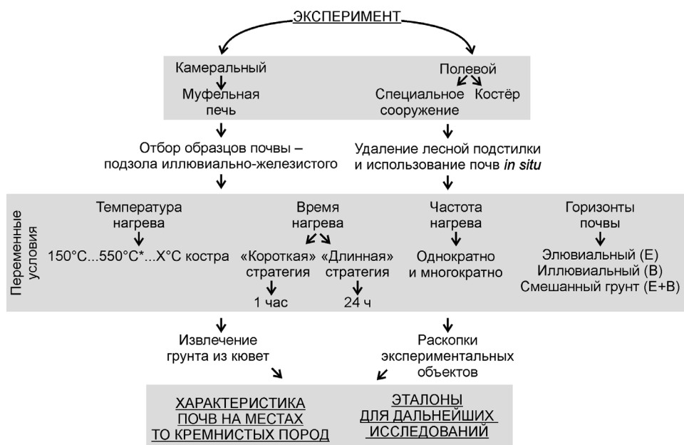
Рис. 2. Дизайн эксперимента по изучению характеристик почв на местах ТО кремня.
