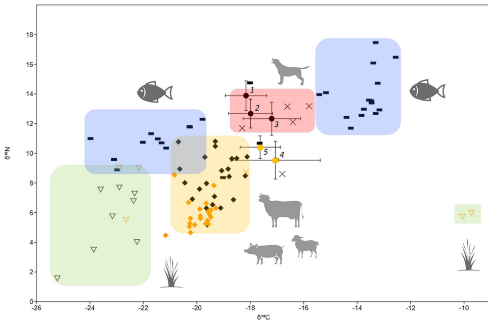
Рис. Распределение изотопных значений \delta^{13}\text{C} и \delta^{15}\text{N} (‰) растений ( \blacktriangledown ), животных ( \blacklozenge и \times ) и рыб ( \times ). Образцы из памятников Боспорского царства обозначены чёрными значками, Херсонеса и его округа – оранжевыми. Усреднённые значения и стандартное отклонение для людей Фанагории эллинистического (1), римского (2), позднеантичного (3) периодов и Херсонеса классического (4) и римского (5) периодов.
